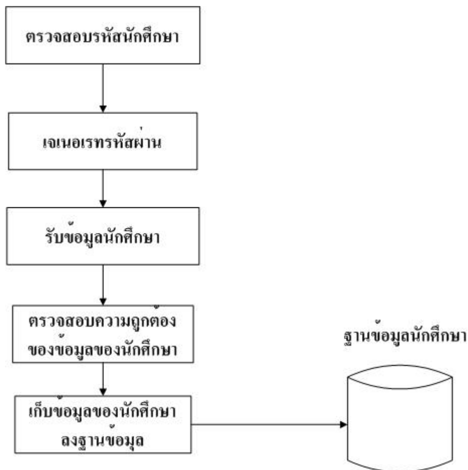
รูปที่ 4-2 หลักการทำงานของระบบลงทะเบียนนักศึกษา
